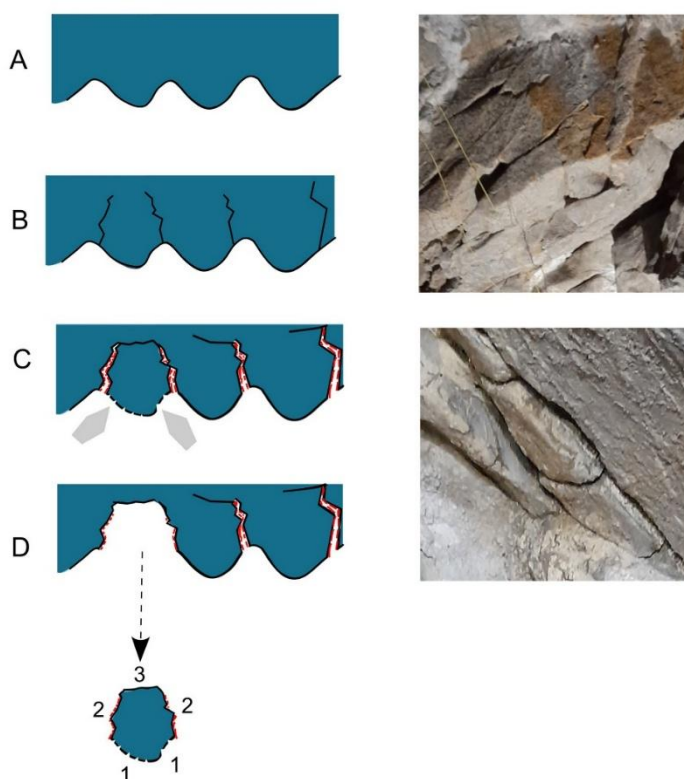
Rekonstrukce vzniku rytého kamenného bloku ze stěny jeskyně Švédův stůl. Schéma znázorňuje praskání a rozpad vápencové stěny, které vedly k oddělení fragmentu; šedě jsou vyznačeny plochy s rytinami. FOTO: Langley, M.C., Škrdla, P., Kmošek, M. et al. Engraved Limestone Block from Švédův stůl Cave, Czech Republic, 2026
